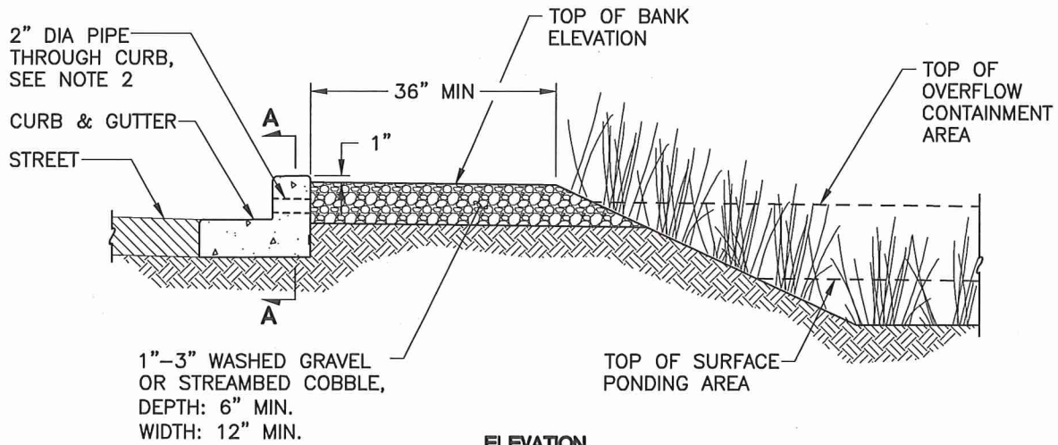
ELEVATION
